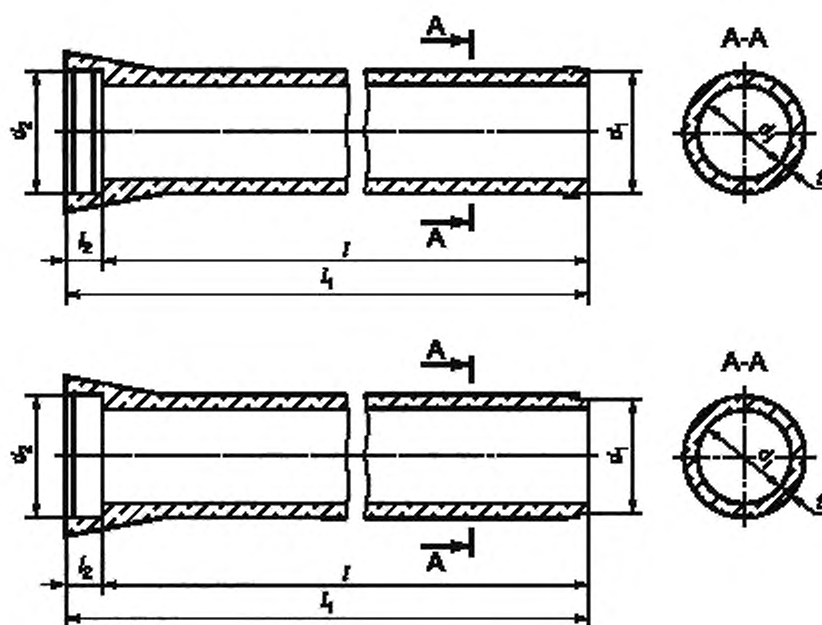
Рисунок А.2 — Общий вид труб типов ТБ и ТС
