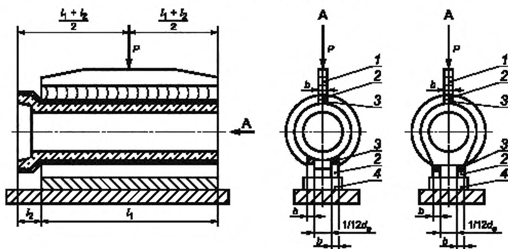
Схемы испытаний труб нагружением
