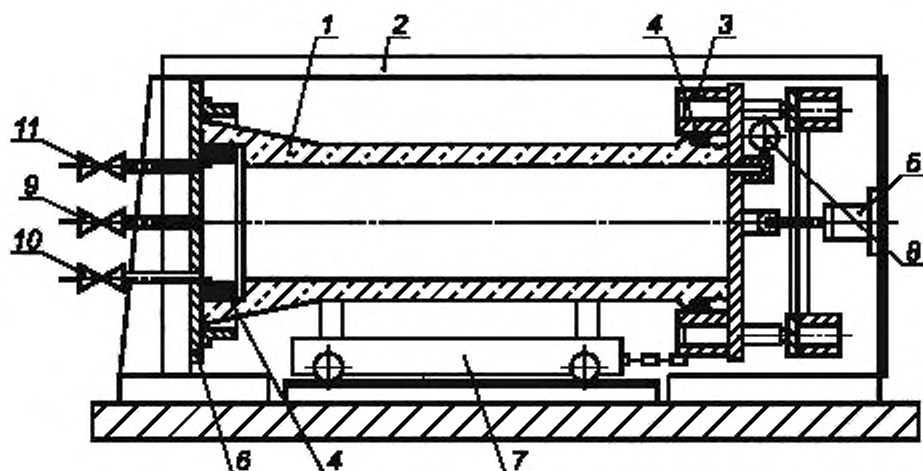
Схемы испытаний труб на водонепроницаемость
