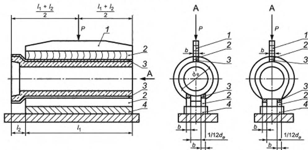
1 — траверса; 2 — деревянные бруски; 3 — резиновые прокладки или цементно-песчаный раствор; 4 — основание
